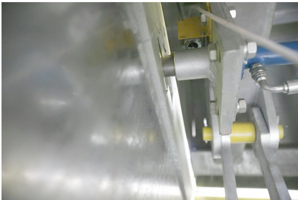
Регулировка фиксаторов в задвинутом положении ВК2-ВК4
