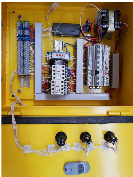
Электрический шкаф
