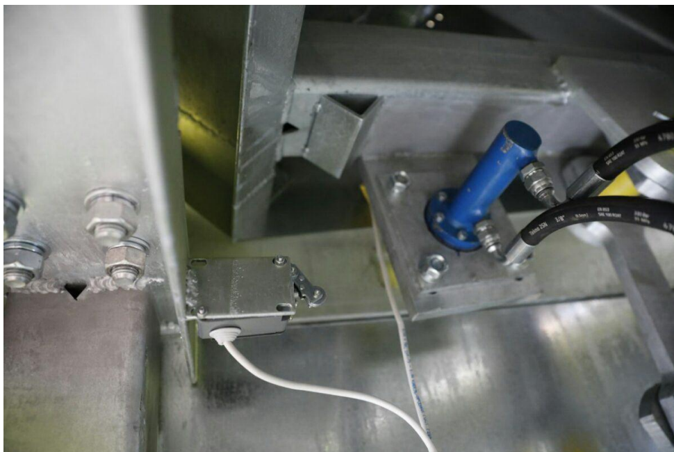
Концевой выключатель нижнего положения гидроцилиндра ВК3
