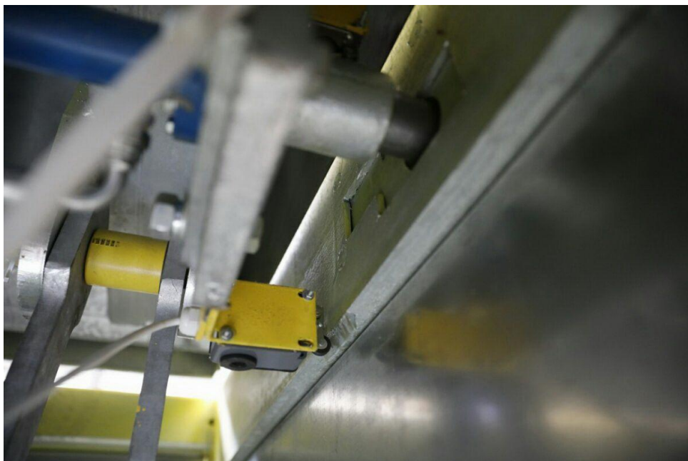
Концевой выключатель верхнего положения гидроцилиндра ВК1
